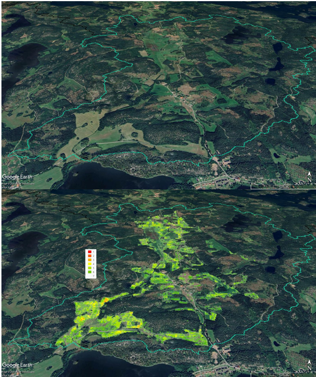
Figur 4. Litet delavrinningsområde i Östergötland, utan (ovan) och med (nedan) beräknade erosionsriskklasser över mobilisering av markpartiklarna i fält.
