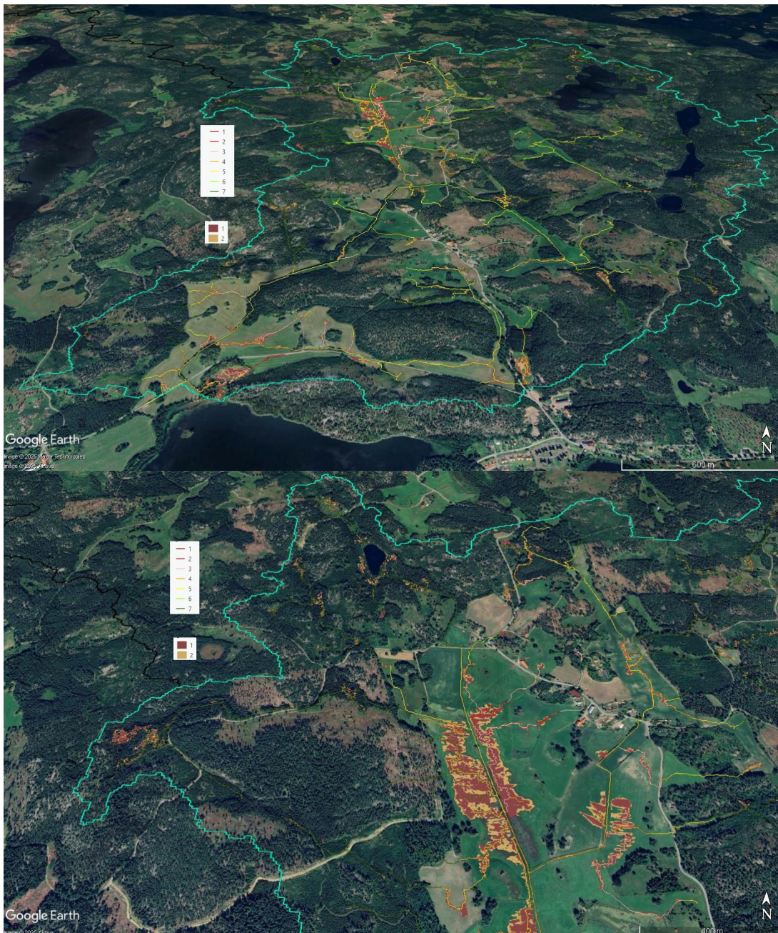
Figur 6. Litet delavrinningsområde i Östergötland med beräknade erosionsriskklasser över flödes- och materialackumulering samt dispergerade flöden, för hela området (ovan), och för det nordvästra hörnet (nedan).
